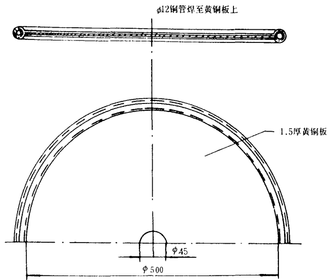
图 A2 保持电极结构图(需画两个)
